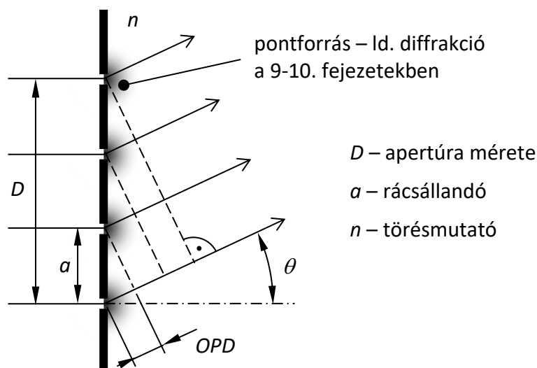
39. ábra. Diffrakciós rács modellezése többhullámú interferencia segítségével.
