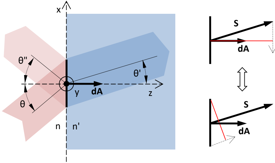
11. ábra. Az elemi felületen áthaladó/visszaverődő síkhullám teljesítményviszonyai leírásánál használt jelölések összefoglalása.
