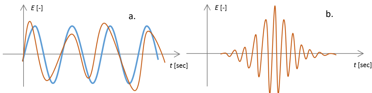
56. ábra. Azonos teljesítményspektrumú hullámok: véletlen kezdőfázisú spektrális komponensek (a), és azonos kezdőfázisú spektrális komponensek (b) esetén.
