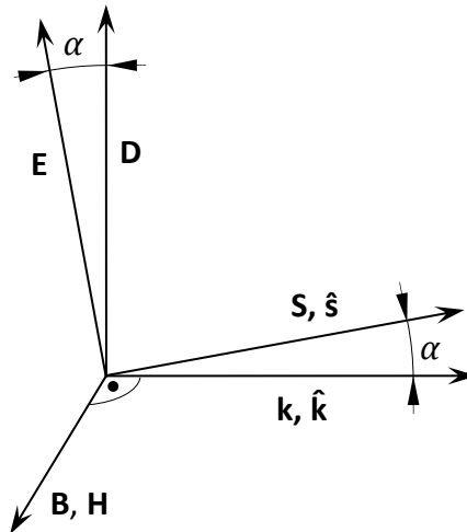
69. ábra. Elektromos/mágneses térerősség-, dielektromos eltolás-, indukció-, hullámszám- és Poynting-vektorok kapcsolata elektromos anizotrópia esetén.
