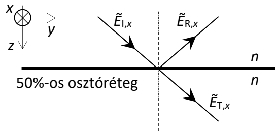
33. ábra. 50%-os osztólemezen áthaladó/visszaverődő síkhullám térampitúdói.
