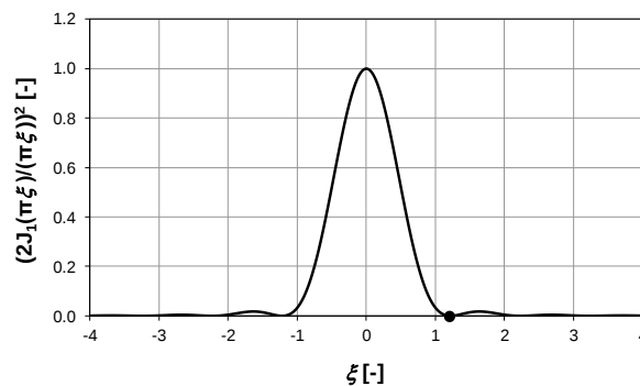
50. ábra. Körapertúra távolféri diffrakciós intenzitáseloszlása.
