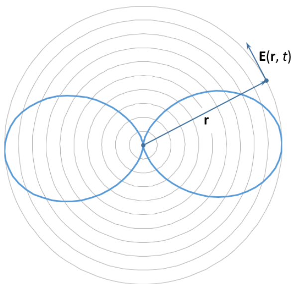
64. ábra. Dipólsugárzó távoltere a hullámfrontok, a polarizáció és az intenzitás-iránykarakterisztika feltüntetésével.
