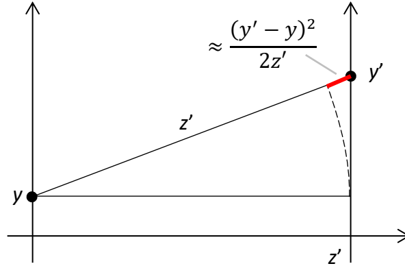
46. ábra. A Fresnel-integrálban szereplő parabolikus hullámfrontok szemléltetése.
