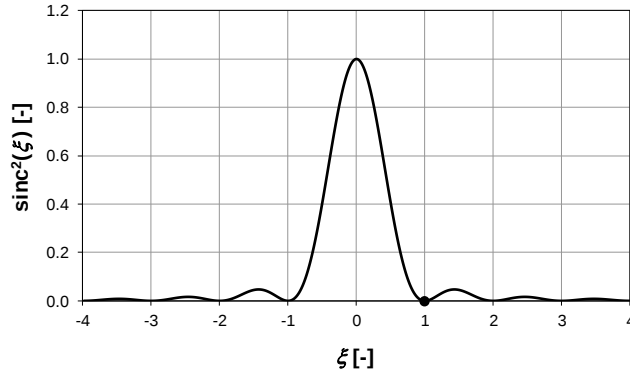
48. ábra. Téglalap-apertúra távolféri diffrakciós intenzitáseloszlása.
