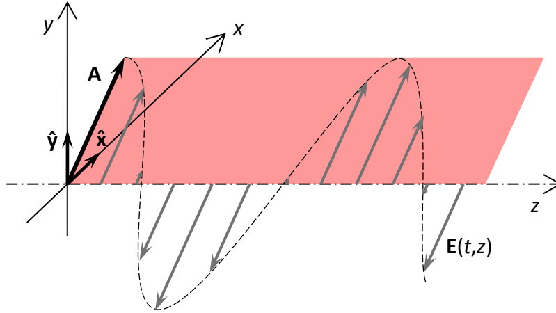
65. ábra. Lineárisan polarizált EM hullám szemléltetése.
