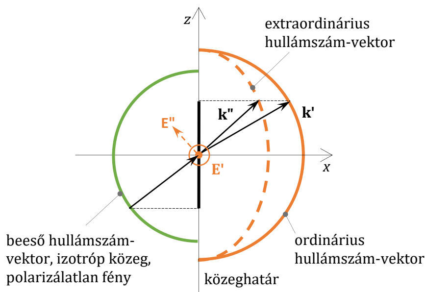
75. ábra. Fénytörés izotróp/anizotróp közeg határán.
