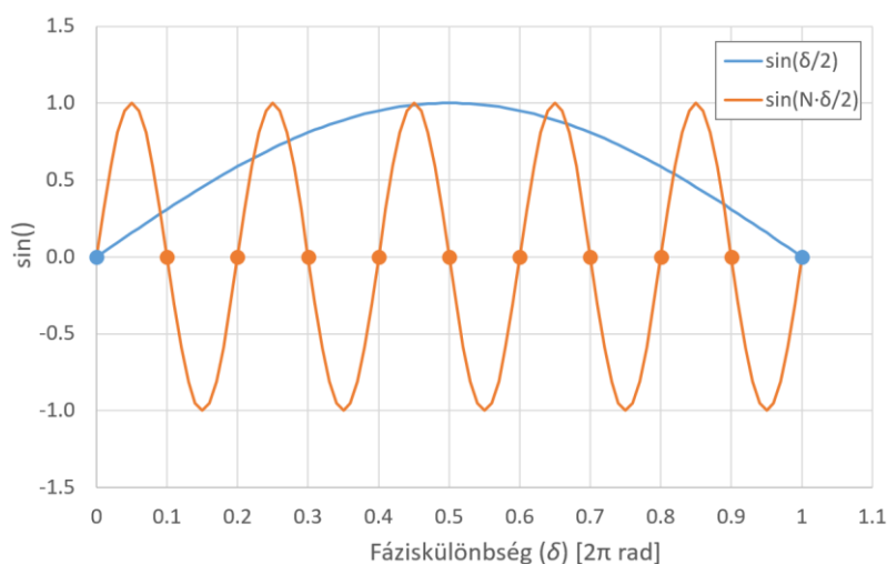
38. ábra. Grafikus szemléltetés a (242) és (243) összefüggések értelmezéséhez.
