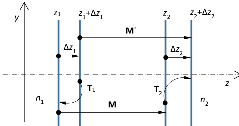
23. ábra. Magyarázat az \mathbf{M}' mátrix felírásához.
