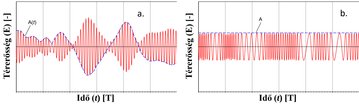
60. ábra. Kaotikus, spontán emissziójú (termikus) (a) és indukált emissziójú fényforrás (b) elektromos térerőssége időfüggésének bemutatása.
